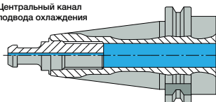
Тип ADB Подвод охлаждения через отверстие или фланец
